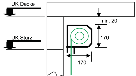
Schnitt B-B
